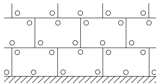
W formos smeigių išdėstymas mineralinės vatos MW-PT atveju
