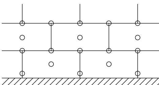
T formos smeigių išdėstymas polistirolu EPS-F atveju
