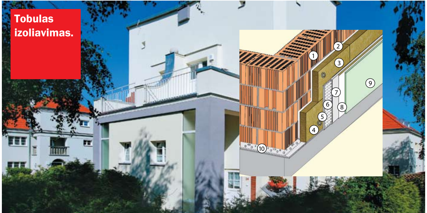
Baumit fasadų apšiltinimo sistema Mineral
